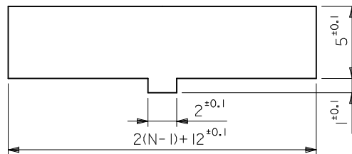
参考パネルスロット寸法 PANEL SLOT DIM.(REF.) (パネル厚: 0.8~2.0) (THICKNESS: 0.8-2.0)
