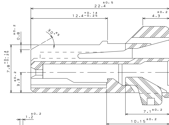
断面 A-A ( 尺 度 5 : 1 )
