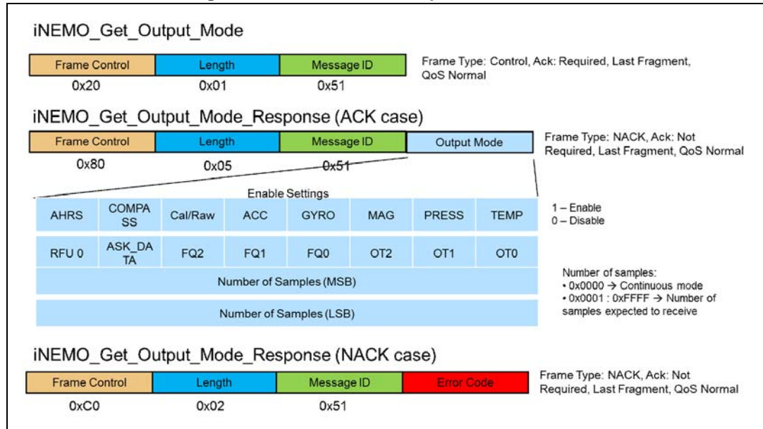
Figure 30. iNEMO_Get_Output_Mode frames
