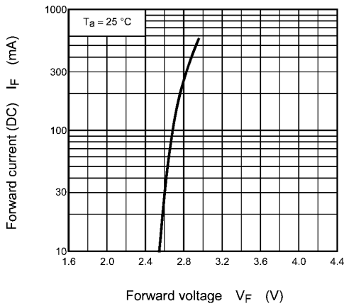
Fig. 8.1 I_F - V_F
