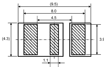
Fig. 10.3.1 (Unit: mm)
